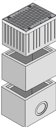
Univerzální odtoková vpust
