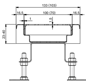
Žlab ZUS
