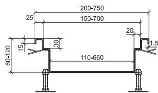
Žlab PZU
