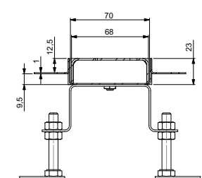
Žlab ZUSI
