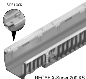
RECYFIX-Super 200 KS
